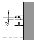
DETAIL UPEVNĚNÍ VODÍCÍCH LIŠT DO OTVORU NA OTVOR
